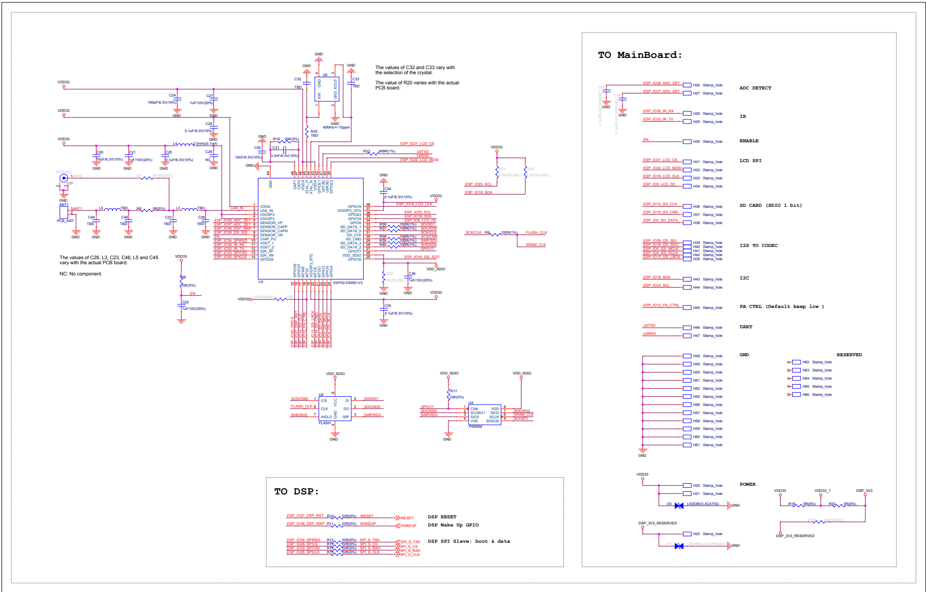
图 5: ESP32-DU1906 模组原理图 (1)
