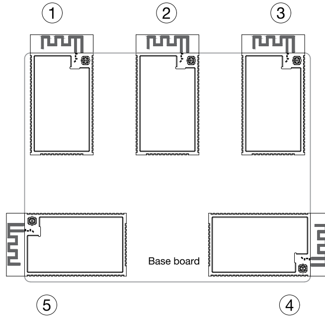
图 15: 模组在底板上的位置示意图
